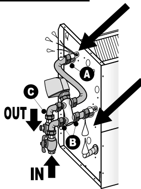
Attacchi idraulici dell'unità ø 1/2" Gas femmina Unit's water connections ø 1/2" Female gas
