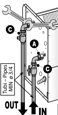
Attacchi idraulici dell'unità ø 1/2" Gas femmina Unit's water connections ø 1/2" Female gas
